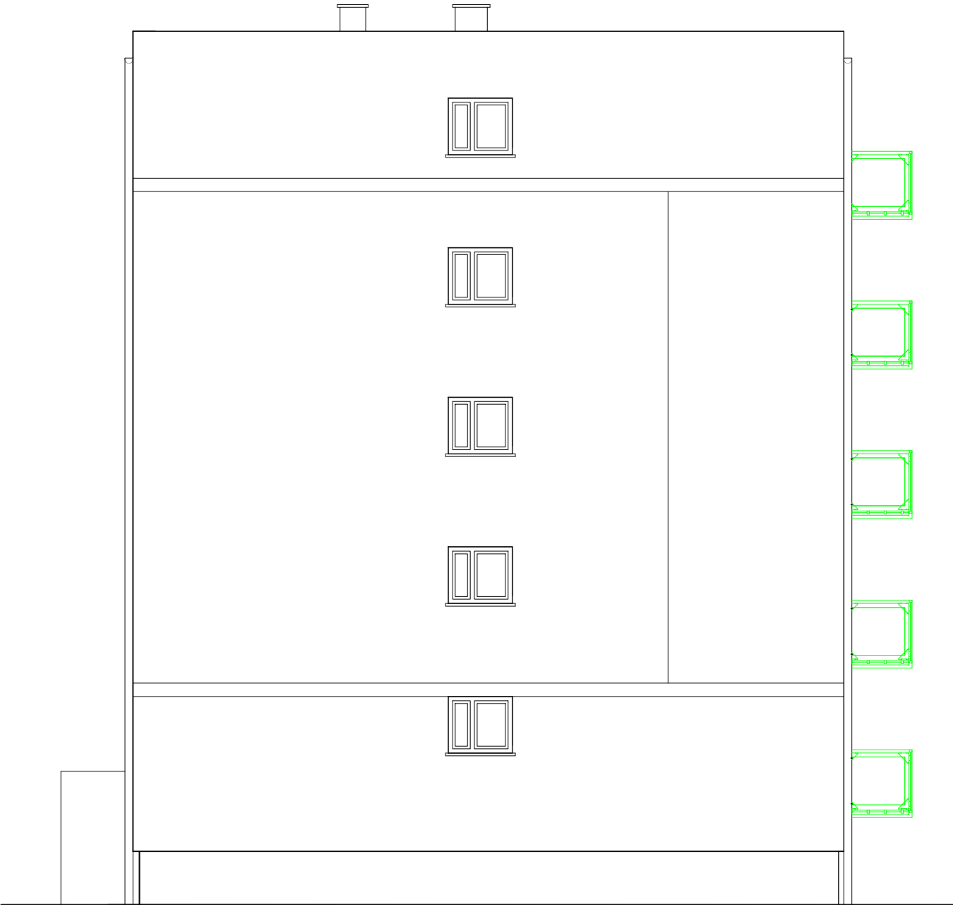
ELEWACJA POŁUDNIOWA
